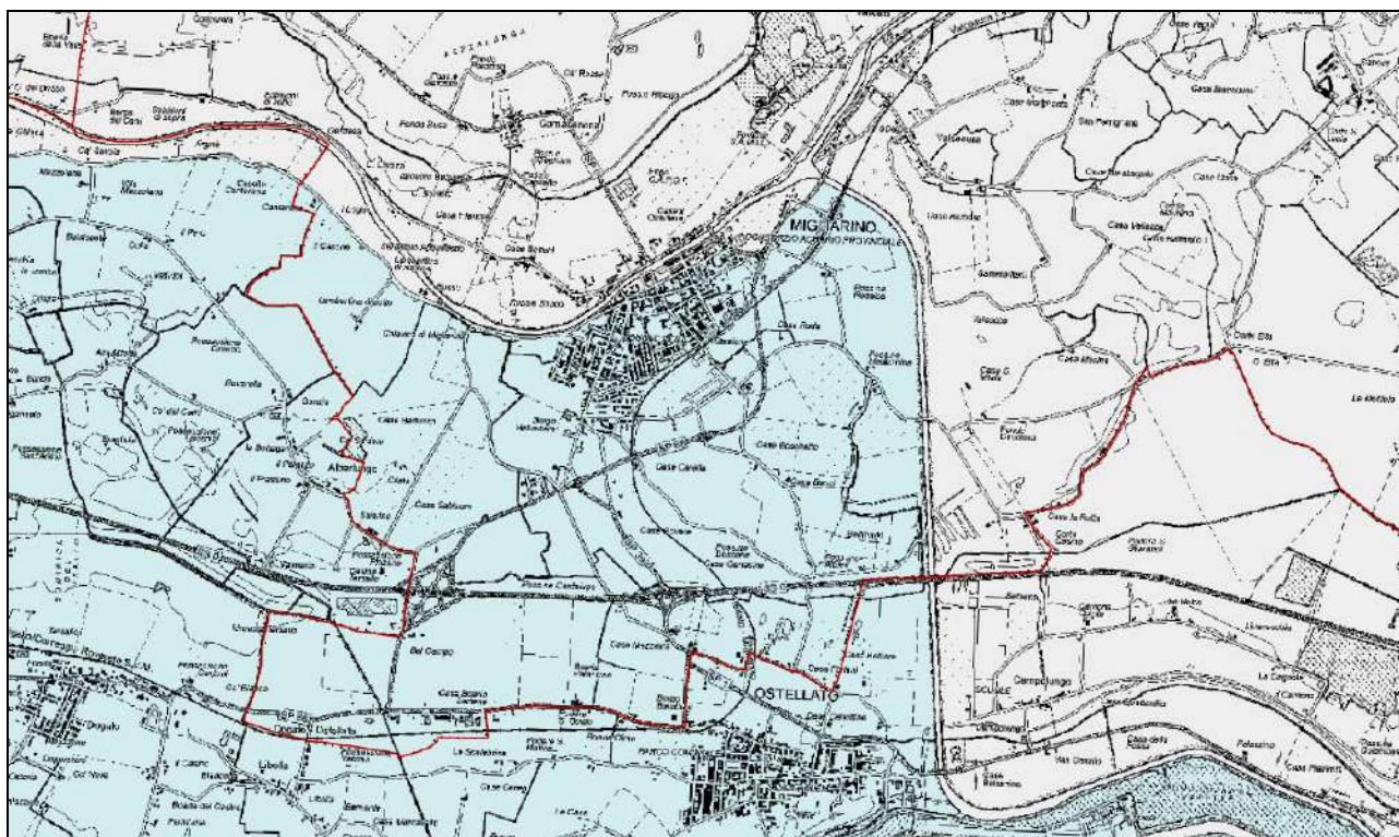
FIGURA 5 – Mappa della pericolosità idraulica da Reticolo Principale di Pianura, zoomata su Migliarino - UoM ITI021-Bacino Reno.
