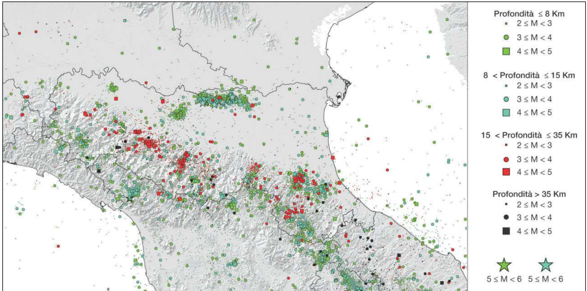
FIGURA 2.20 - mappa degli epicentri verificatisi nella Regione Emilia Romagna, raggruppati in funzione della profondità degli ipocentri, ovvero la suddivisione è per sismi verificatisi a profondità inferiore a 8 km, per profondità comprese tra 8 e 15 km, per profondità comprese tra 15 e 35 km e per profondità maggiori di 35 km.
