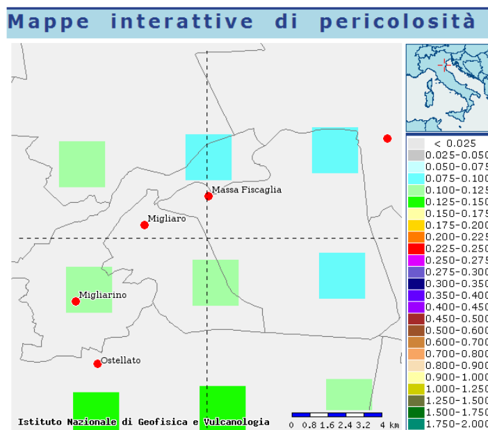
FIGURA 2.26 – Carta pericolosità sismica, da progetto DCP – INGV – S1. fonte: http://esse1-gis.mi.ingv.it
