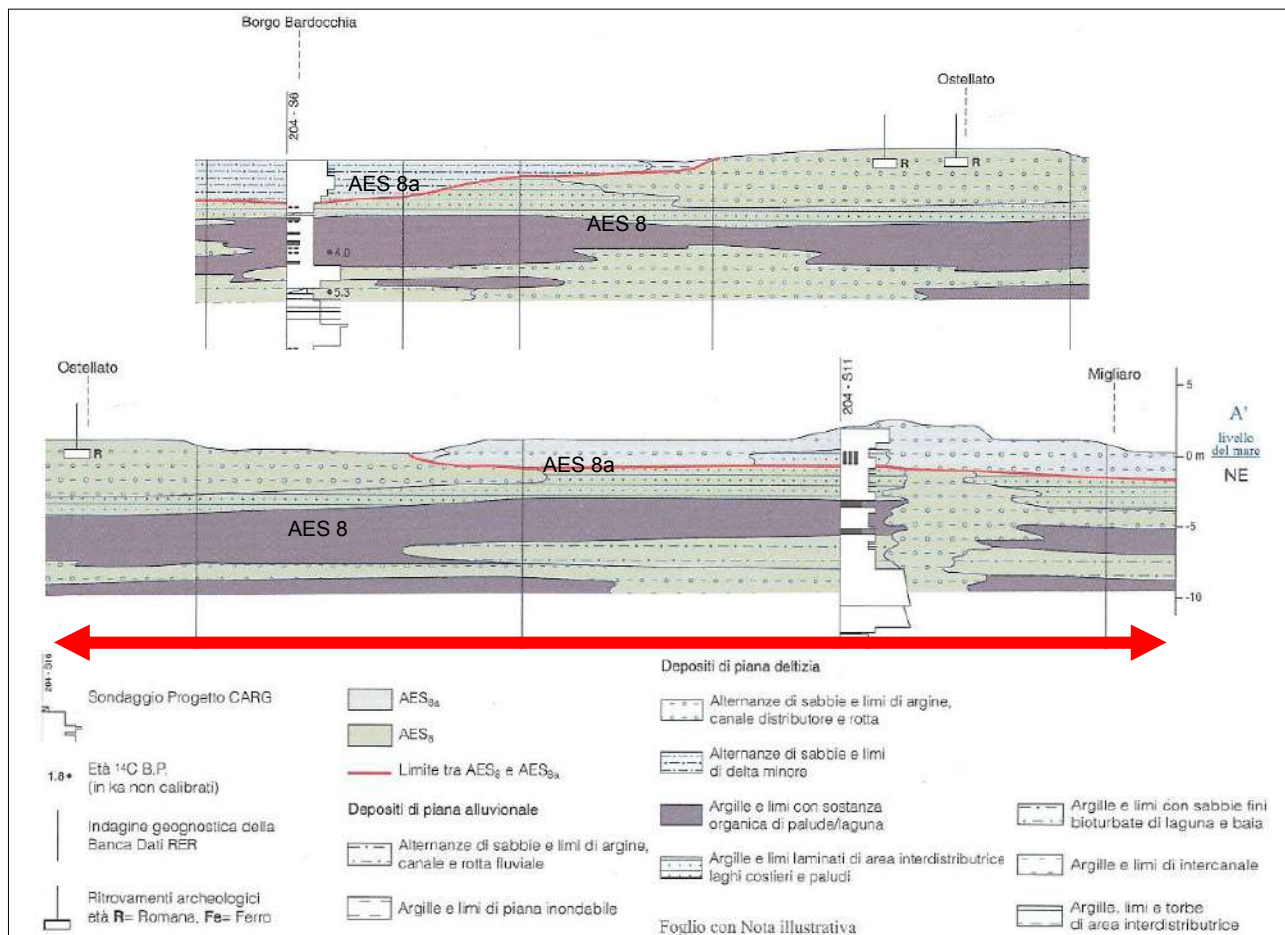
FIGURA 5.10 - Sezione geologica compresa tra Ostellato e Migliario. Viene aggiunta anche la porzione di sezione compresa tra Borgo Bardocchia e Ostellato, poiché qui sono visibili anche le datazioni con il C14 di alcuni livelli geologici. ( http://www.isprambiente.gov.it/Media/carg/204_PORTOMAGGIORE/Foglio.html )
