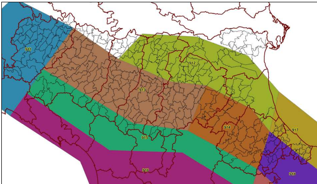
FIGURA 2.10 - Aree sismogenetiche in Emilia Romagna
