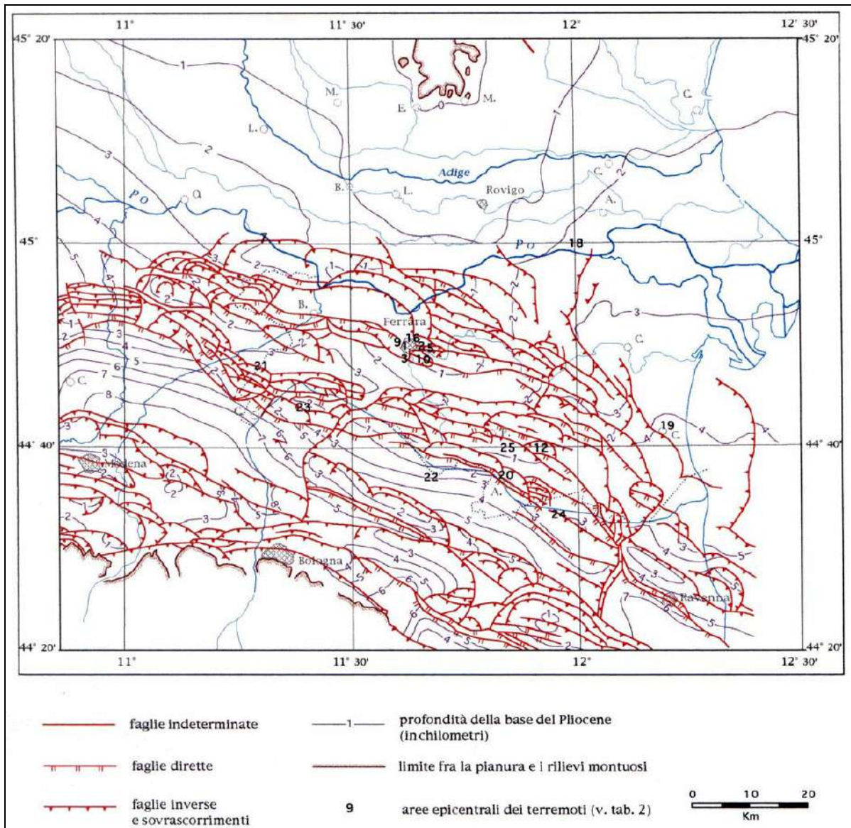
FIGURA 2.3 – Carta strutturale della Pianura Padana orientale (Pieri e Groppi, 1981, CNR, 1992)
